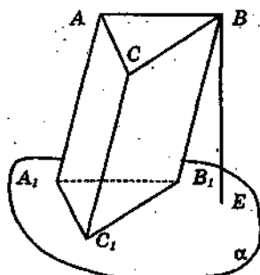
Наклонная призма BE — высота призмы
