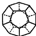
Додекаэдр
