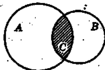
C = A \cdot B Рис. 80
