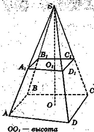
OO_1 — высота
