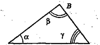
\alpha, \beta, \gamma — углы треугольника
