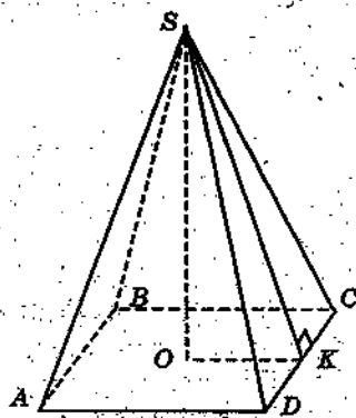
SK — апофема
